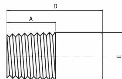
ANSI B16.11
