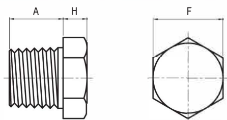
ANSI B16.11
