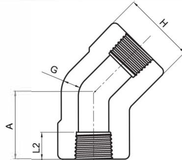
2000# (mm) ANSI B16.11
