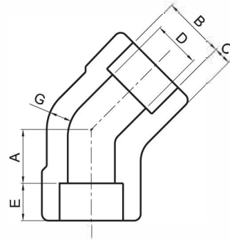
3000# (mm) ANSI B16.11
